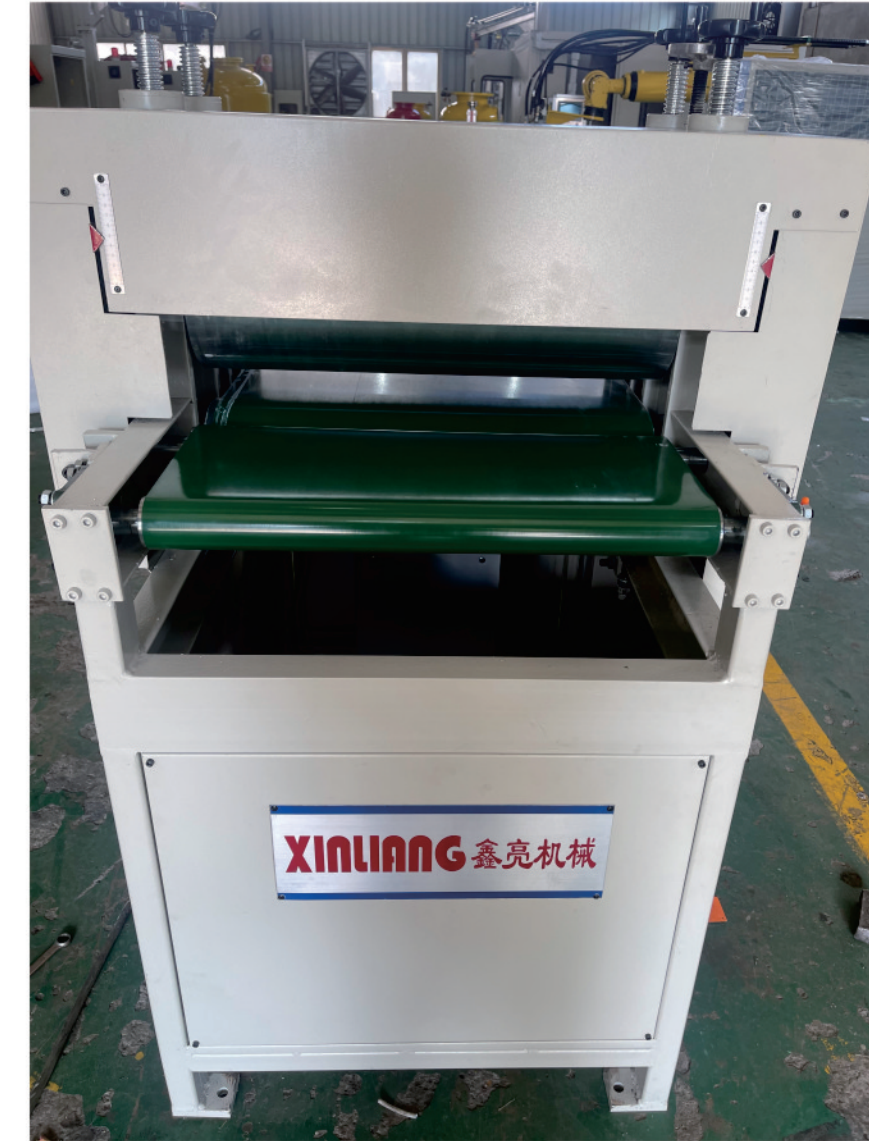
压泡机 Bubbler
